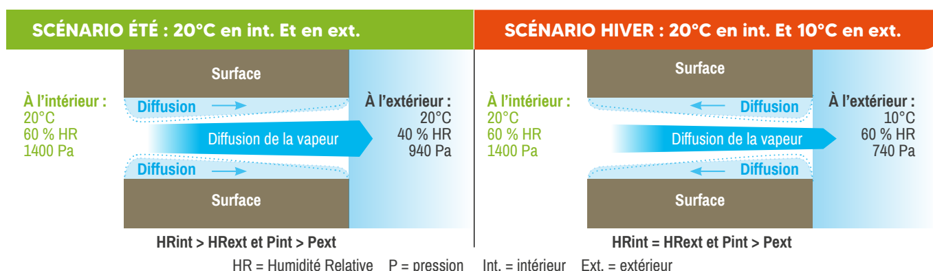
Figure 22 - Diffusion de la vapeur d'eau à travers la paroi
