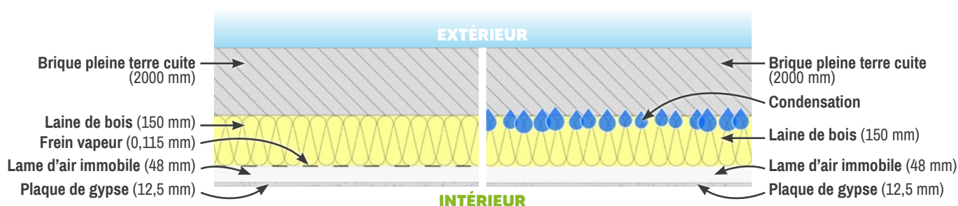
Figure 23 - Paroi brique rénovée avec une solution d'ITI avec (gauche) et sans (droite) mise en oeuvre d'un frein-vapeur - Source : ubakus.com / CODEM
