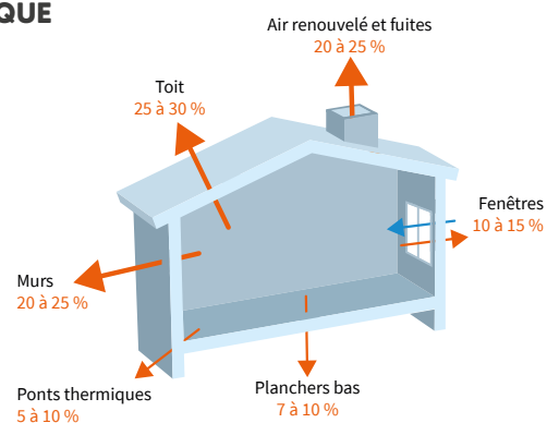
Figure 6 - Répartition des déperditions énergétiques pour une maison construite avant 1974 et non isolée Source : Guide pratique « Isoler sa maison » de l'ADEME
