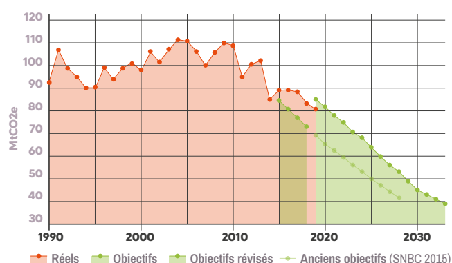
Figure 10 - Emissions globales de GES du secteur du Bâtiment par rapport aux objectifs fixés par la SNBC Source : Observatoire Climat-Energie
