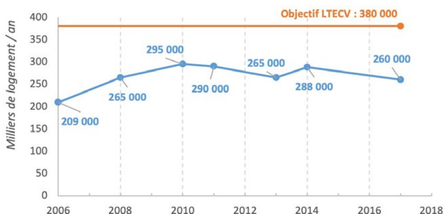
Figure 11 - Evolution du nombre de rénovation performante ou très performante - Source : CODEM, TREMI / OPEN
