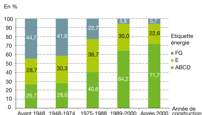
Figure 5 - Répartition des étiquettes énergie DPE dans les résidences principales par période de construction - Source : Commissariat général au développement durable [2]
